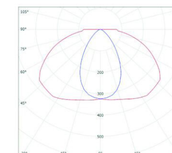
配光曲线图
