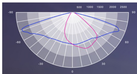
配光曲线图 Light Pattern
