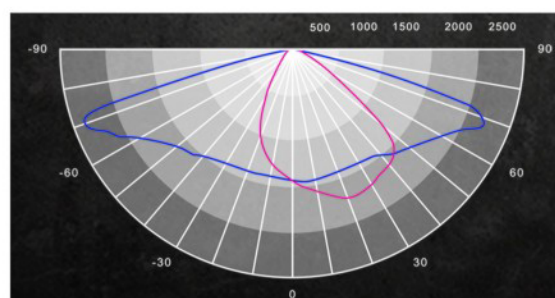
配光曲线图 Light Pattern
